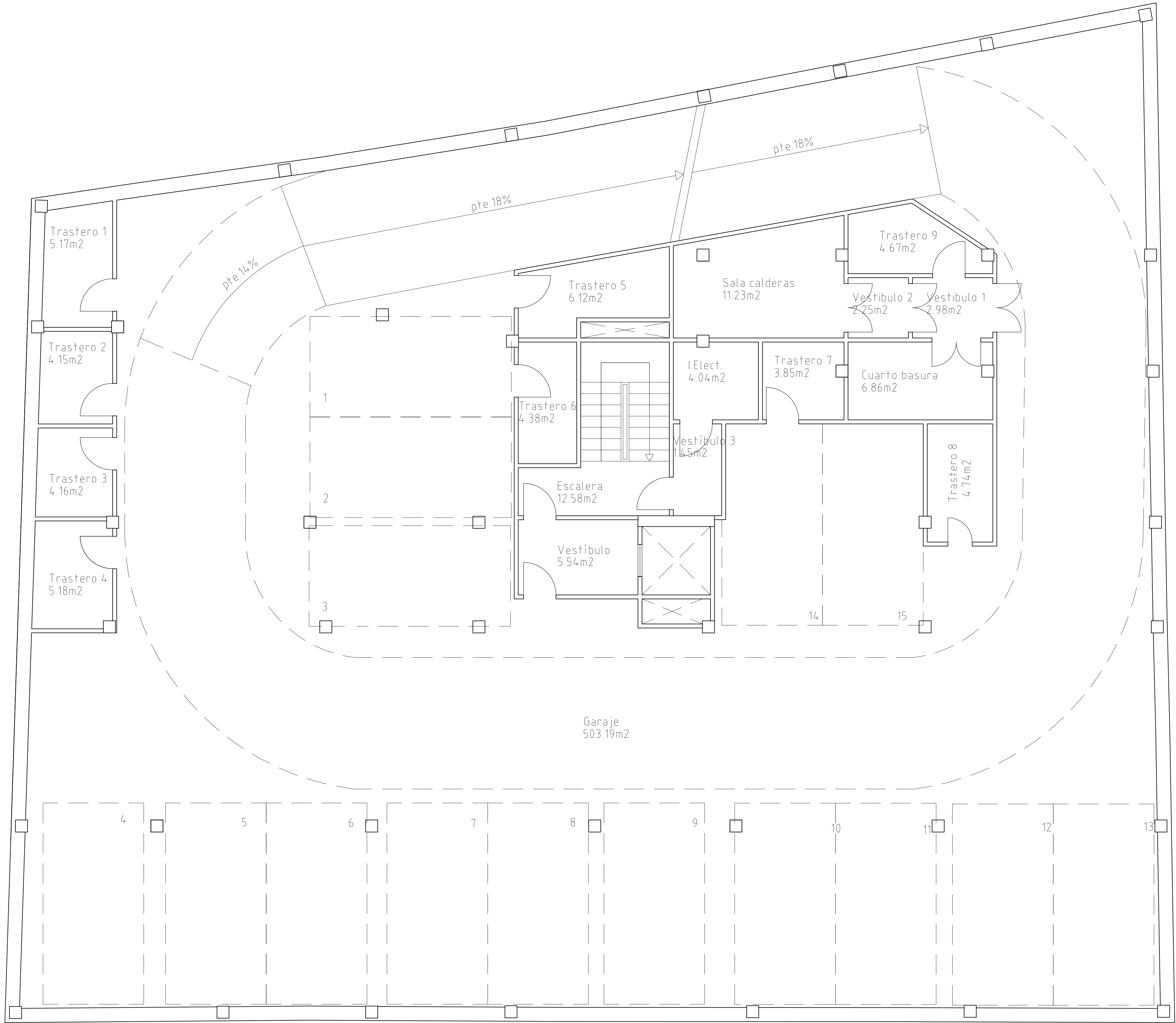
Planta Sótano 1
