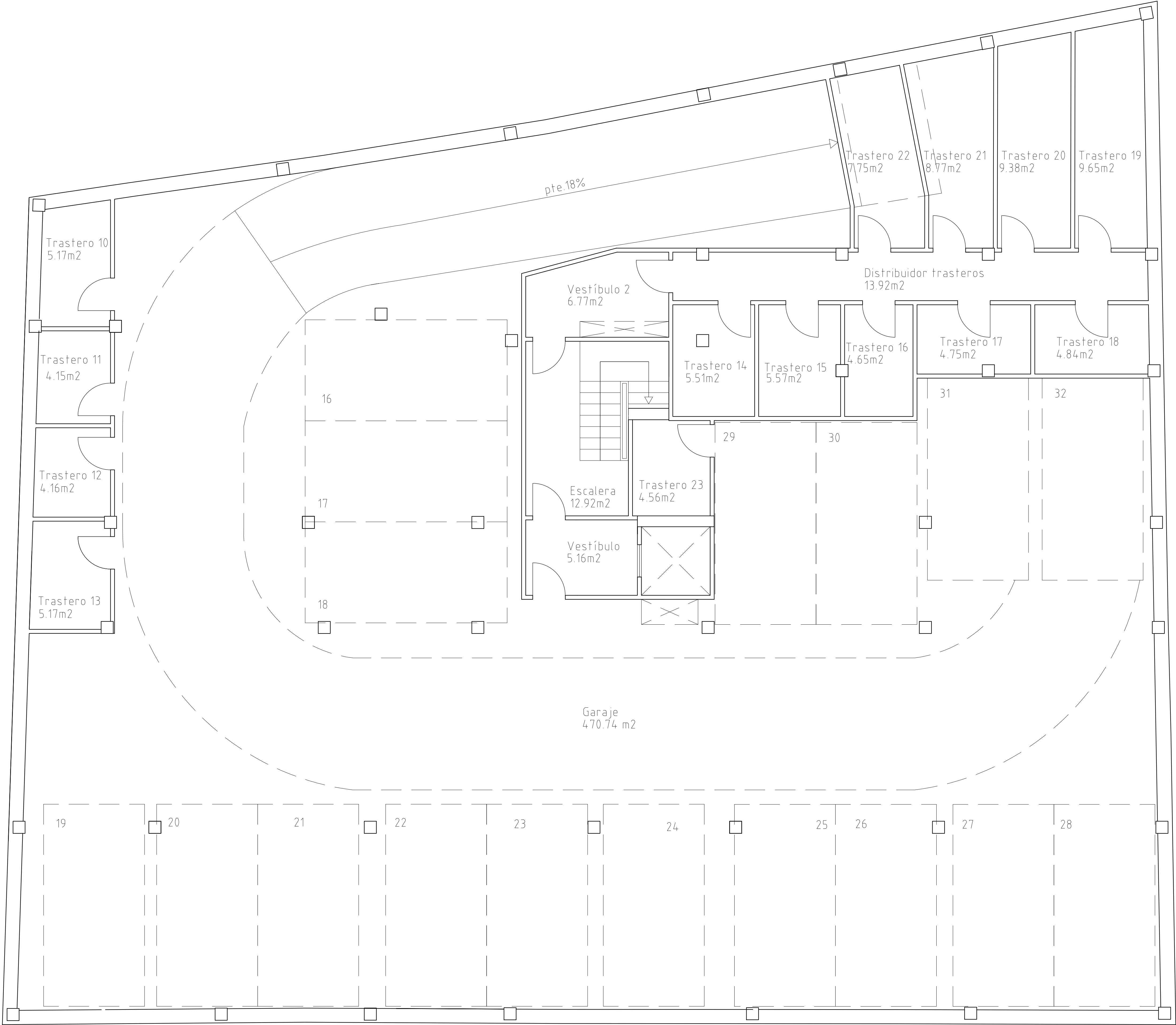
Planta Sótano 2
